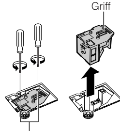
Befestigungsschrauben
